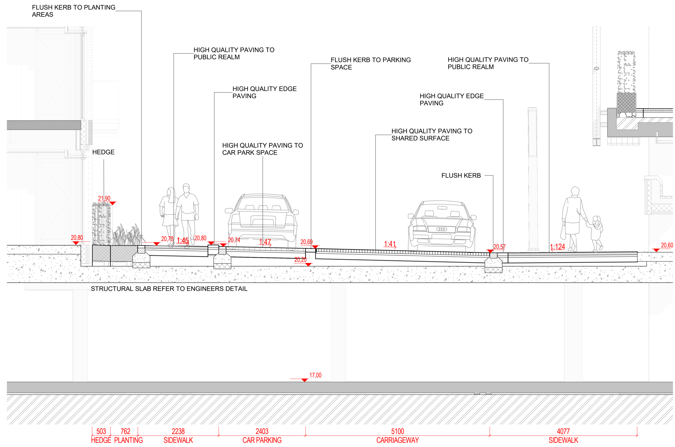
1 SECTION 20 1:50 @A1
